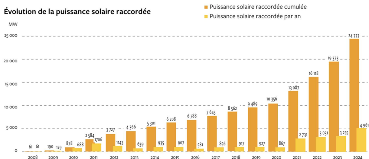
Figure 11 - Évolution de la puissance photovoltaïque raccordée entre 2008 et juin 2024 (source : RTE, Panorama de l'électricité renouvelable 2024)
