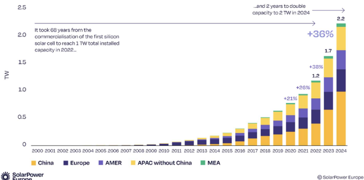
Figure 6 – Puissance totale cumulée entre 2000 et 2024 (source : SolarPower Europe, Global Market Outlook for Solar Power 2025-2029)
