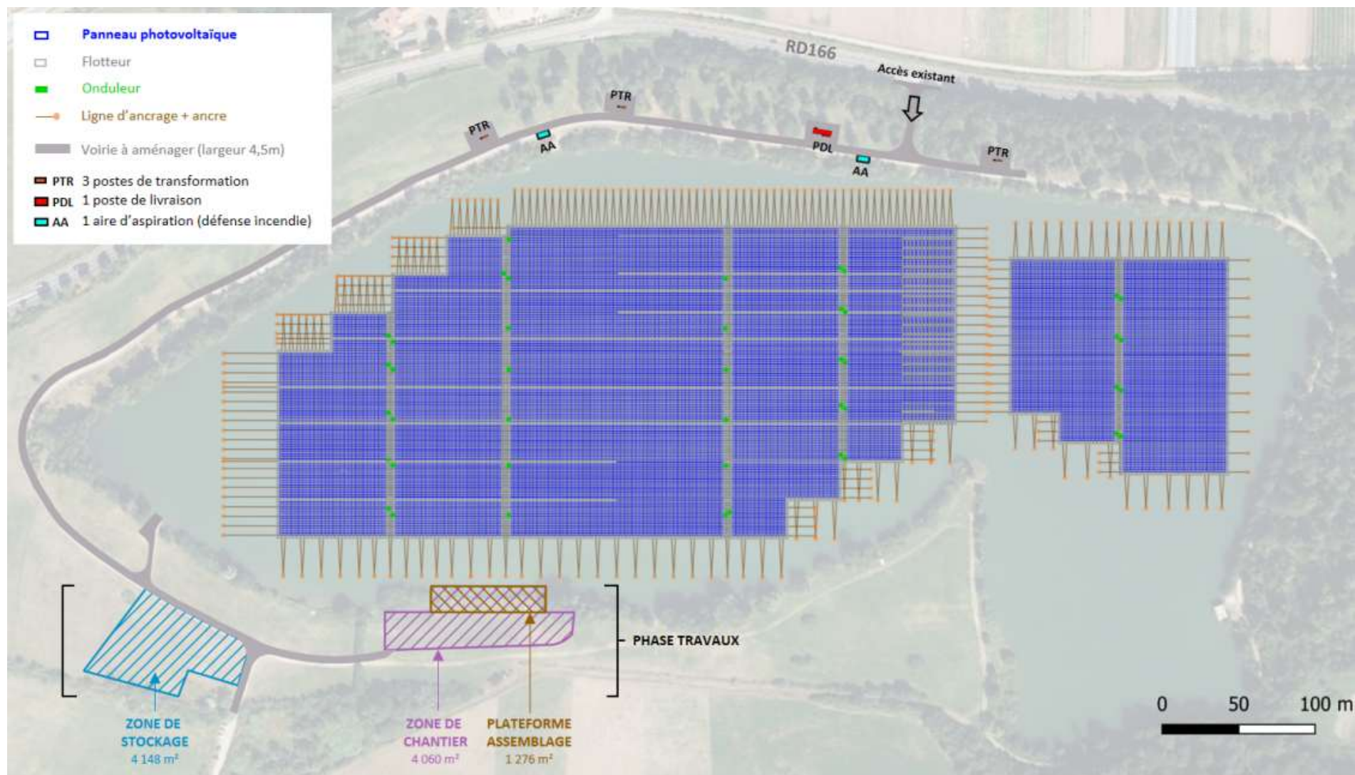
Figure 3 – Plan masse du projet de centrale photovoltaïque flottante de Burnhaupt-le-Bas (source : Étude d'impact, Laketricity)
